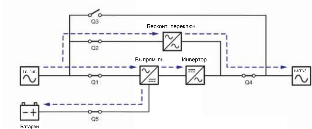
Рисунок 3-5: Схема ESO-режима, подключение одного ИБП к одной линии
